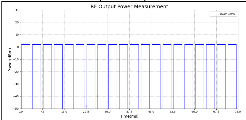
Test_Graph_BR_HOP_NA_1Mbps_Power_NT
